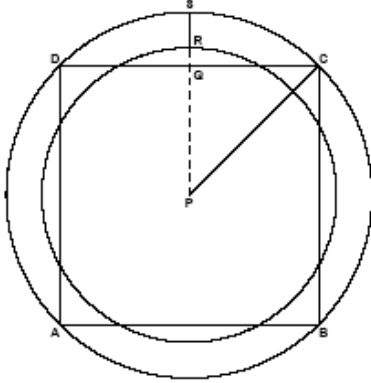
Рис. 1. Построение в «Баудхаяна шульба-сутре»
