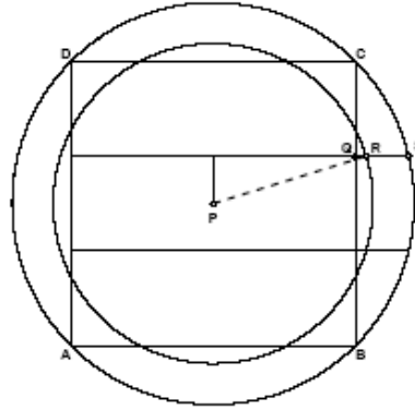
Рис. 2. Построение в «Манаса шульба-сутре»
